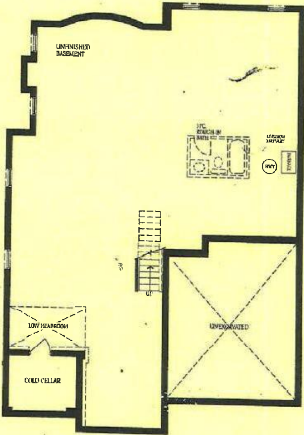
BASEMENT PLAN 'B'
