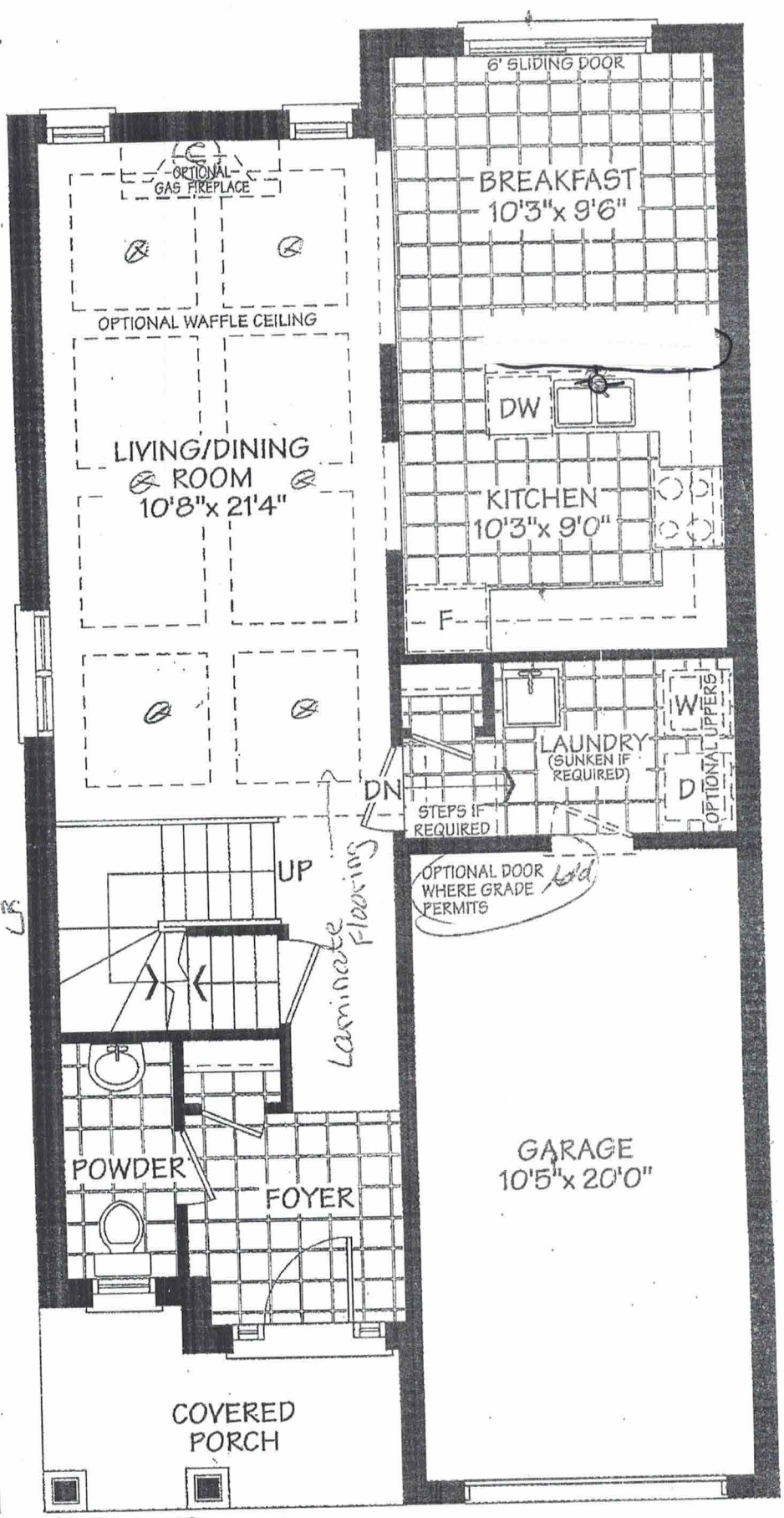
ELEV - B
