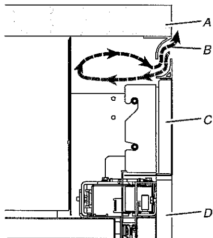
A. Soffit B. Airflow
