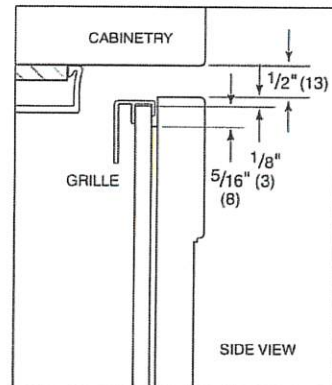
Grille Top
