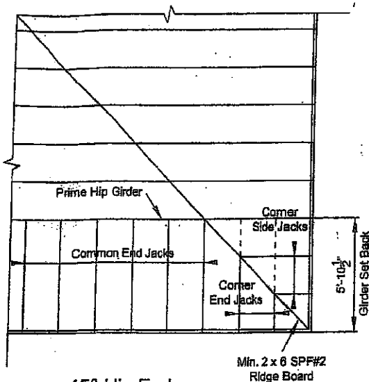
45° Hip End
