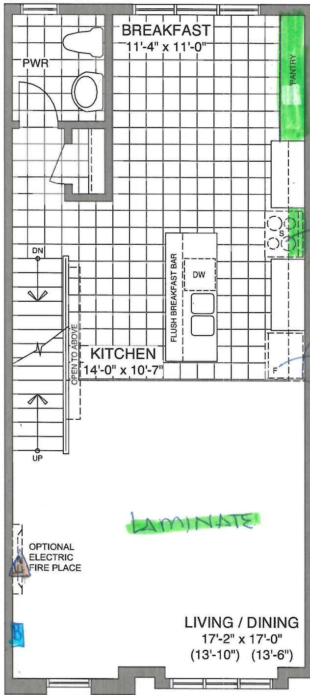
MAIN FLOOR - ELEV A1 & A4
