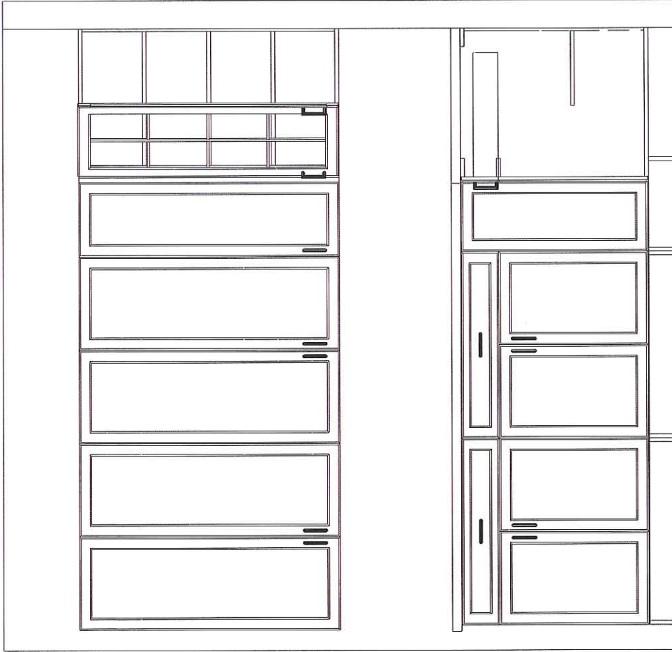
ELEVATION 2
