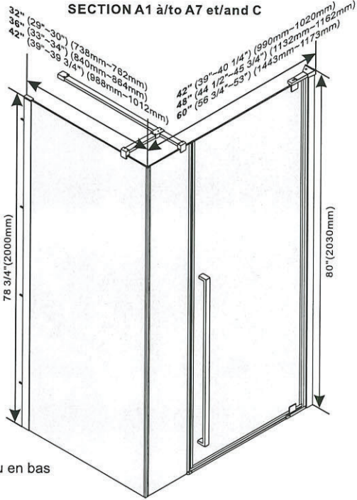
SECTION A1 à/to A7 et/and C
