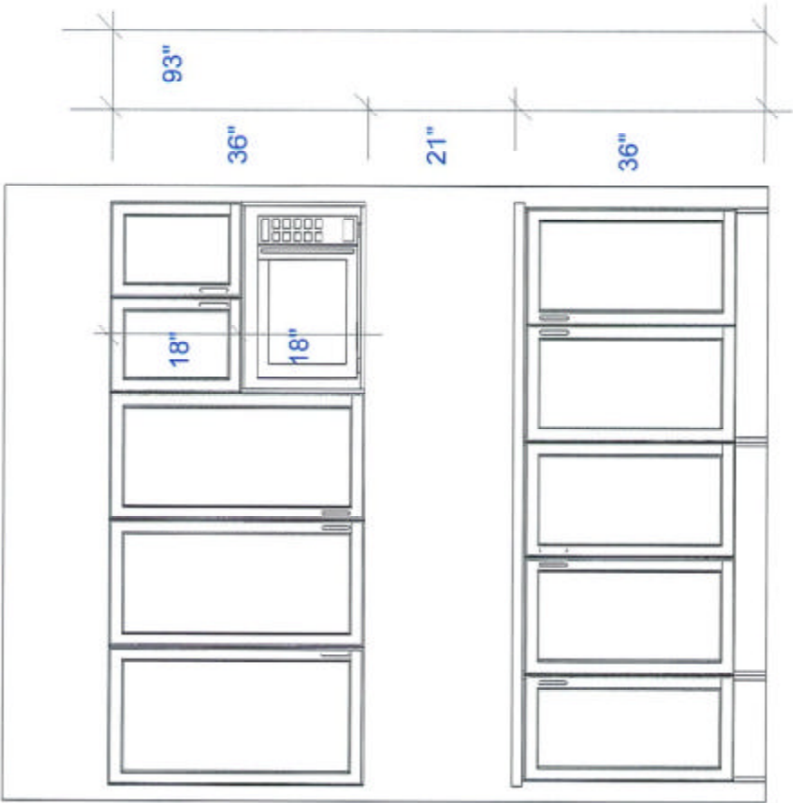
MW WALL ELEVATION
