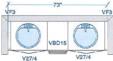
ENSUITE 3
