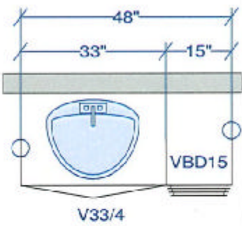
2ND ENSUITE
