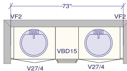
ENSUITE 4
