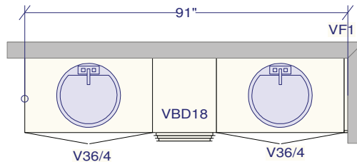
ENSUITE 1
