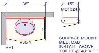
ENSUITE BEDROOM 4
