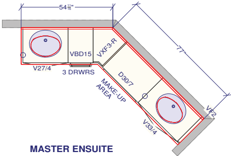
MASTER ENSUITE
