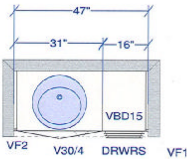
2ND. ENSUITE
