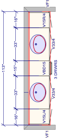
BEDROOM 5 - JACK & JILL ENSUITE
