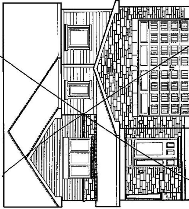
ELEVATION A
