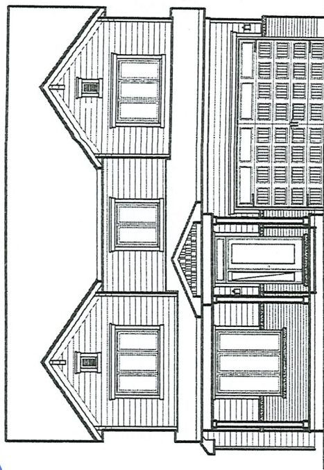
ELEV. 'C'
