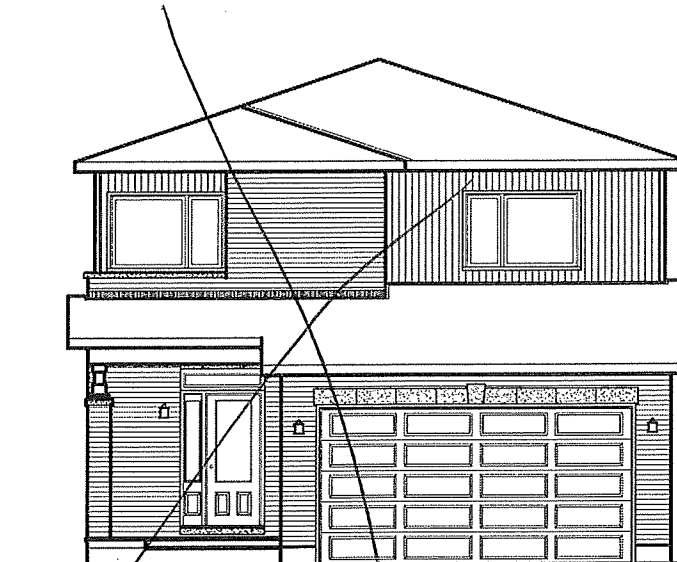
ELEVATION B
