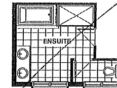
OPTIONAL 5PC ENSUITE ELEVATION A
