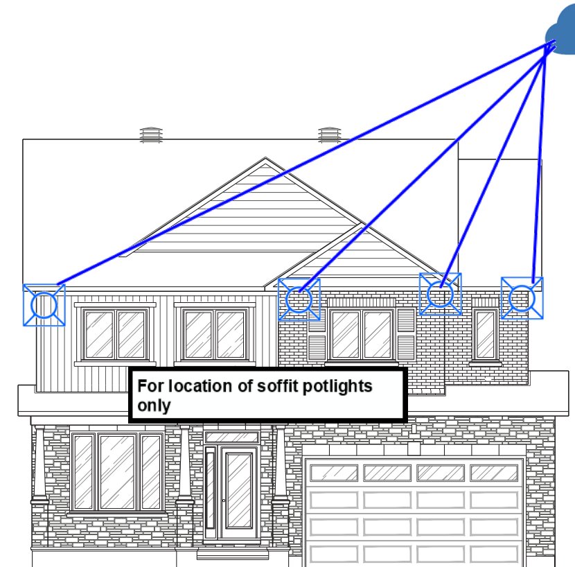
ELEVATION A
