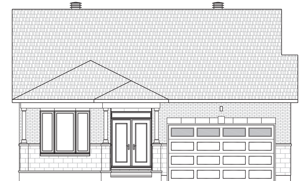
ELEVATION A
